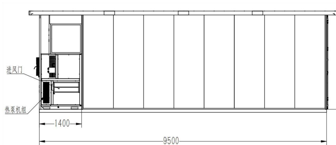
图2 移动烤房右侧视图
