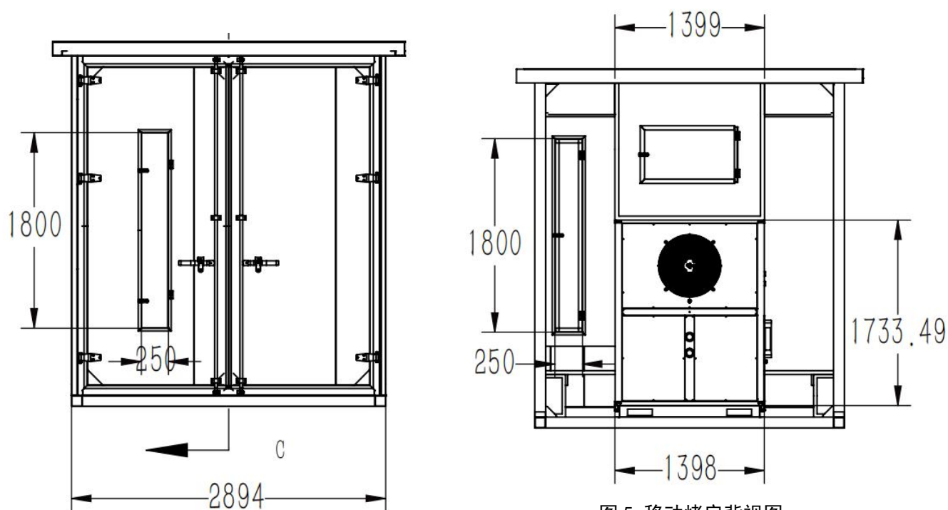
图 5 移动烤房背视图
